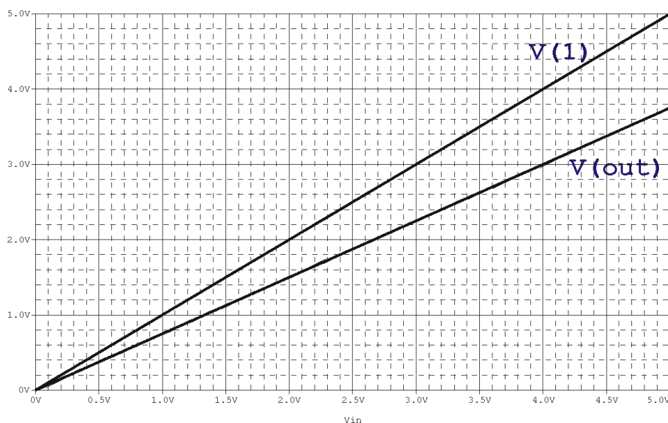
Rys. 7. Wyniki symulacji stałoprądowej układu z rys. 6.
