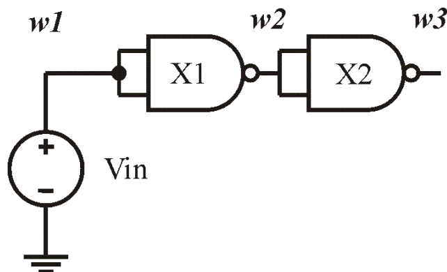
Rys. 14. Schemat połączenia dwóch bramek NAND z rys. 13 w celu zbadania czasu propagacji bramki X1.
