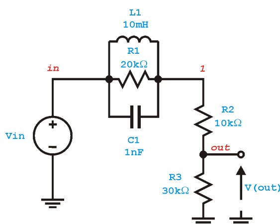
Rys. 6. Prosty układ pasywny poddany symulacji stałoprądowej. Czcionką pochyłą zapisano zastosowane nazwy węzłów połączeniowych.
