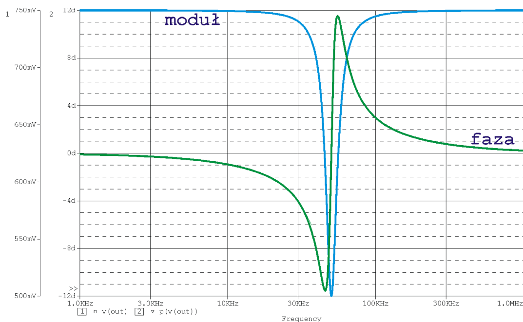
Rys. 9. Wynik symulacji małosygnałowej częstotliwościowej układu z rys. 6. Wykreślony został moduł i faza napięcia w węźle out .
