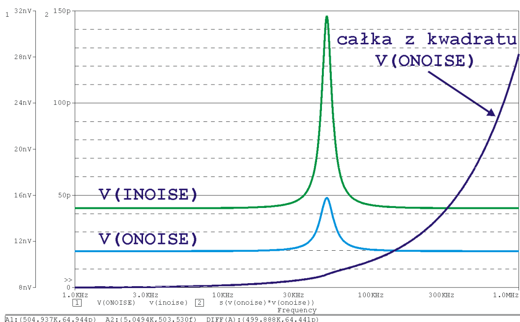
Rys. 12. Wynik symulacji szumowej układu z rys. 6. Wykreślono gęstość widmową napięcia szumów na wyjściu V(ONoise), gęstość widmową napięcia szumów odniesioną do wejścia V(INoise) oraz całkę z kwadratu sygnału V(ONoise).
