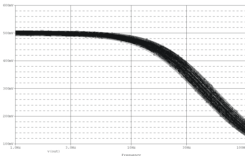
Rys. 17. Wyniki symulacji Monte Carlo układu z rys. 16.
