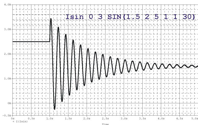
Rys. 5. Przykład deklaracji przebiegu czasowego typu SIN.
