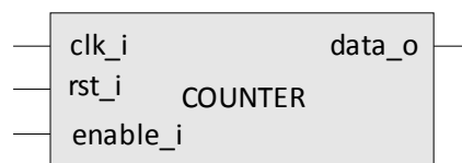
Rys. 39 Blok entity w języku VHDL
