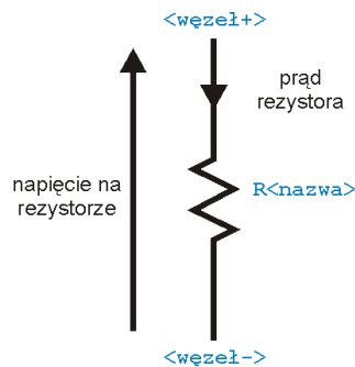
Rys. 1. Elementy z dwoma wyprowadzeniami – zasada pomiaru napięcia i prądu oraz nazewnictwo węzłów na przykładzie rezystora.
