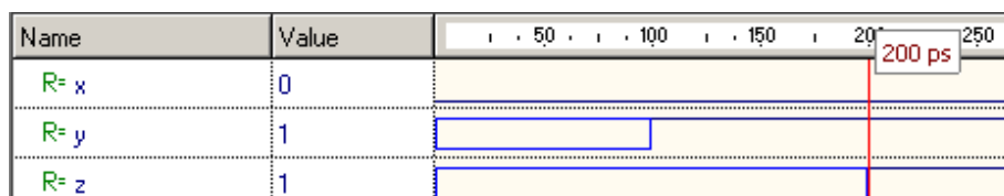
Rys. 33. Wynik działania przykładu z przypisaniem typu blocking .
