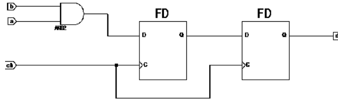
Rys. 36. Wynik syntezy przykładu z przypisaniem typu nonblocking .
