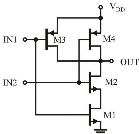
Rys. 13. Schemat bramki NAND CMOS. Węzeł pomiędzy drenem M1 a źródłem M2 nazwany został „10”. Należy przyjąć wymiary wszystkich tranzystorów równe W=0,9\text{ }\mu\text{m} L=0,6\text{ }\mu\text{m} , podłoża tranzystorów typu p należy podłączyć do węzła vdd a podłoża tranzystorów typu n do masy.
