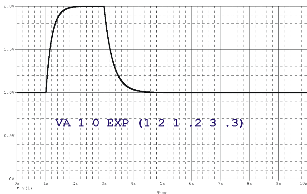
Rys. 3. Przykład deklaracji przebiegu czasowego typu EXP.
