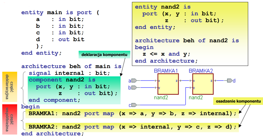
Rys. 40. Przykład osadzenia komponentu.
